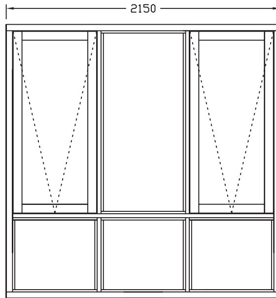
FTW 2100 X 2150 A
