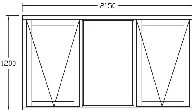
FTW 1200 X 2150 A
