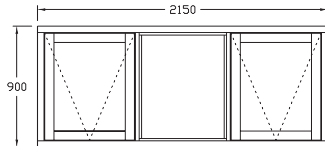
FTW 900 X 2150 A
